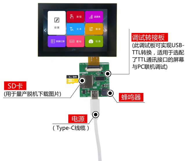
图 1-3 调试工具图
