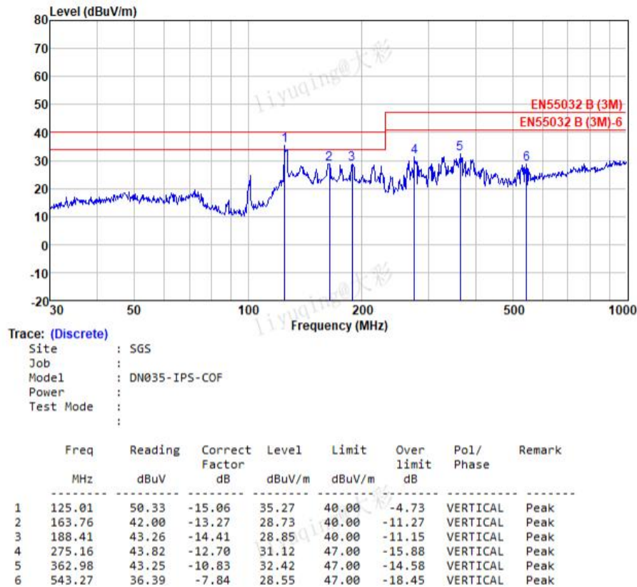
图 5-7 RE 测试垂直方向
