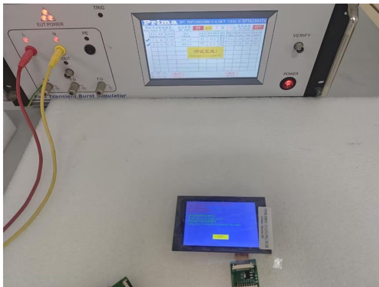
图 5-3 EFT 测试图
